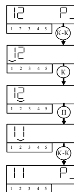
Редактирование служебных параметров (изменение типа реакции на НС Ј, со 2 на 1 во втором контуре)
